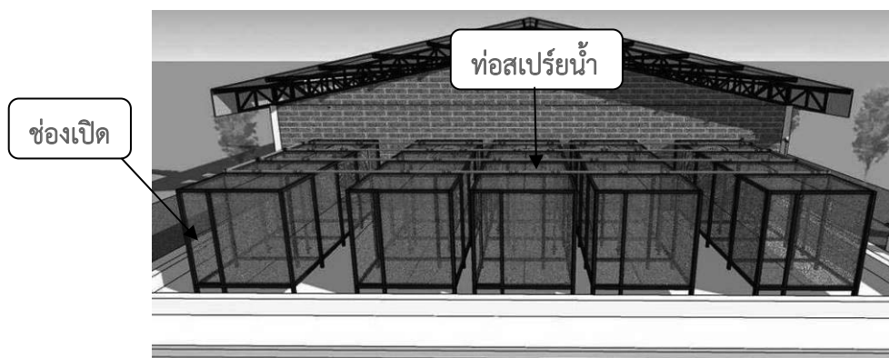
รูปที่ 7.3-9 ม่านกระจายน้ำกำจัดกลิ่นหลังพัฒมโรงเรือน
