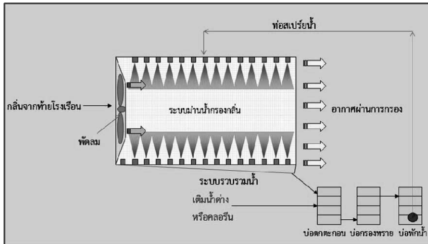
รูปที่ 7.3-5 แสดงขั้นตอนการทำงานของระบบกรองกลิ่นหลังพัฒน์แบบม่านกระจายน้ำ
