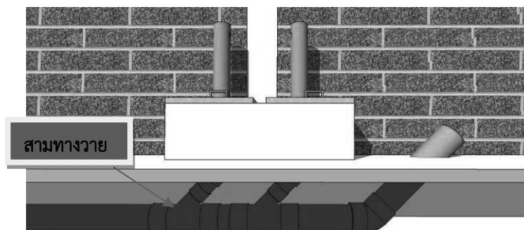
รูปที่ 6.1-7 ติดตั้งสามทางรูปตัววายสำหรับจุดโค้งของท่อ
