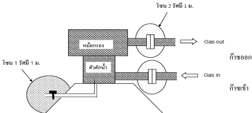
รูปที่ 8.2-7 การจัดแบ่งโซนเครื่องดักน้ำและหม้อกรองติดตั้งด้านก่อนเข้าเครื่องเพิ่มความดัน
