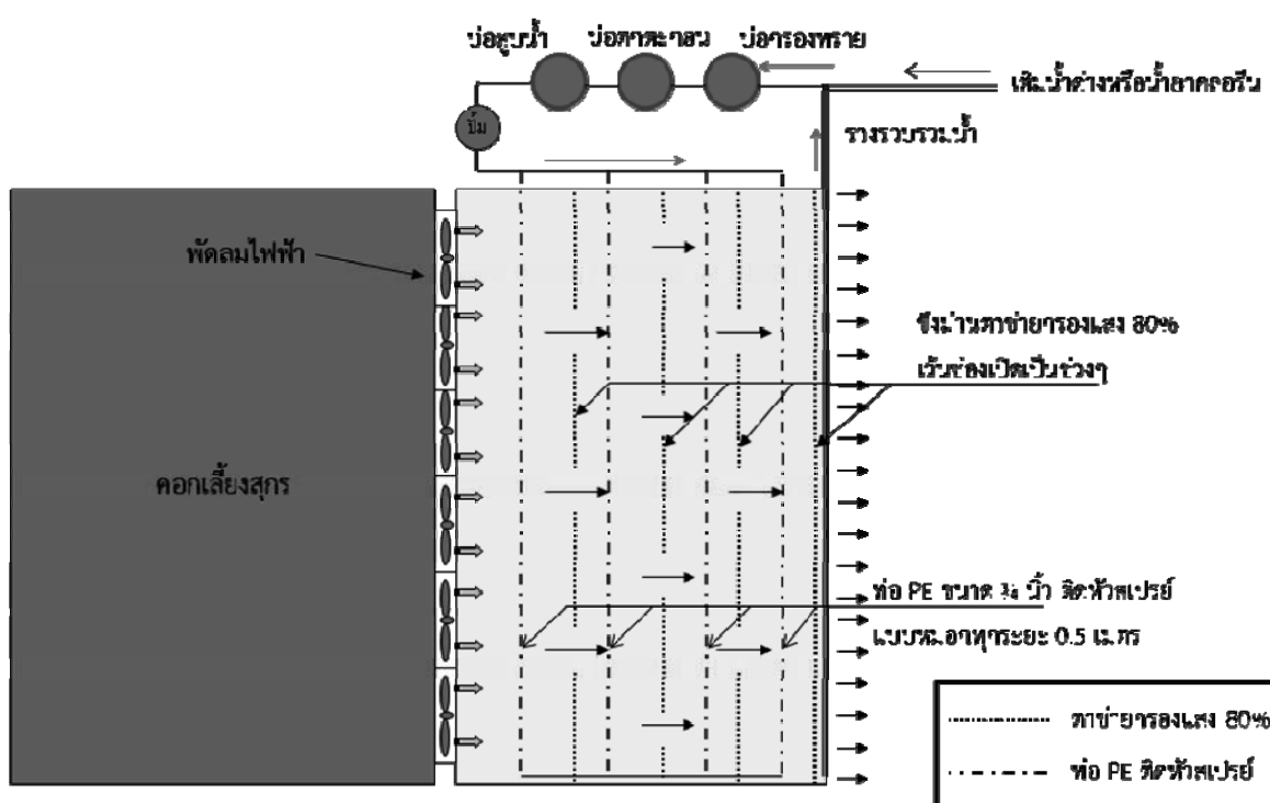
รูปที่ 7.3-17 แสดงขั้นตอนการทำงานของระบบรอกลิ้นแบบมาน้ำเต็มพื้นที่
