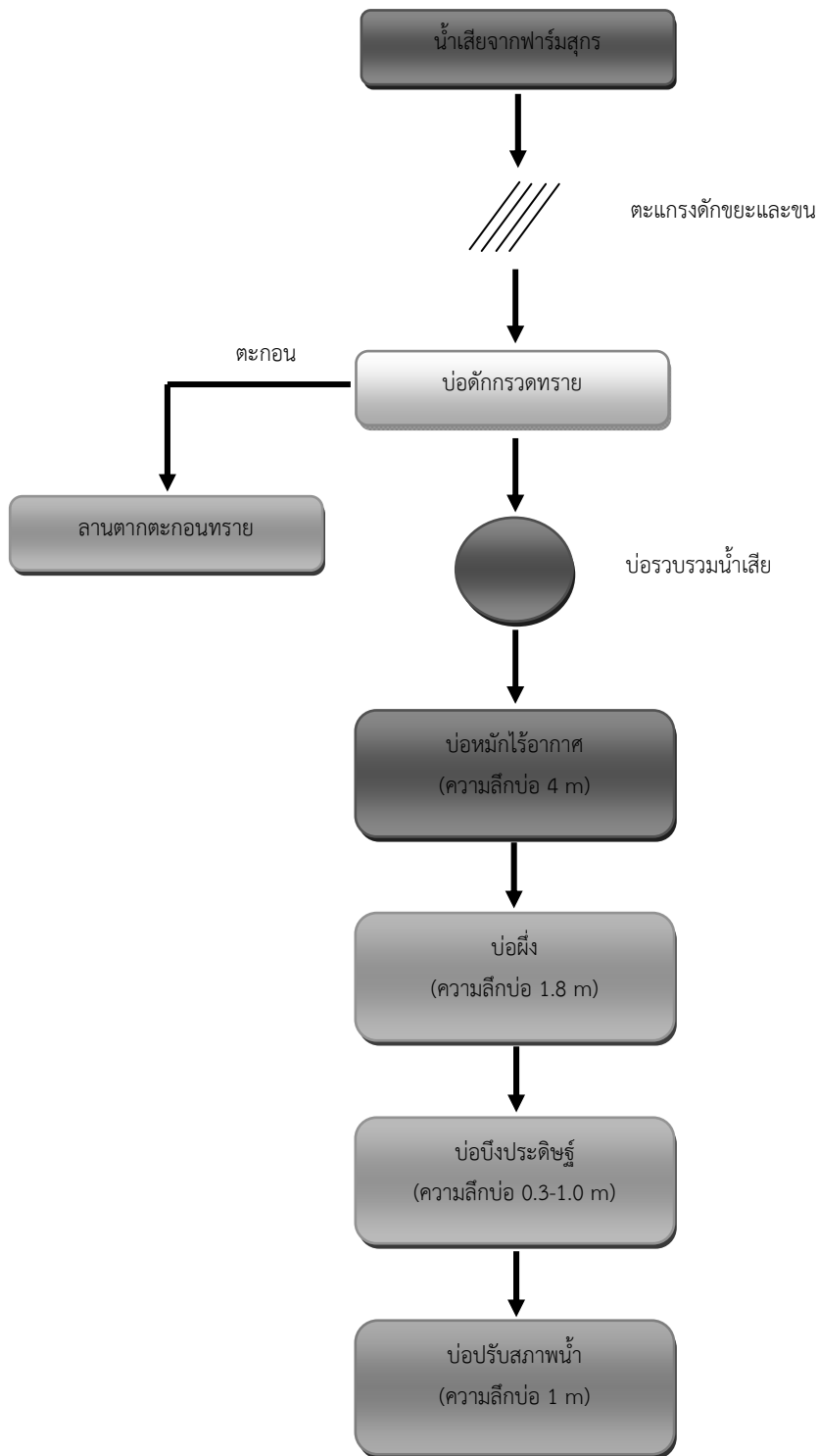
รูปที่ 6.4-5 กระบวนการบำบัดน้ำเสียแบบบ่อหมักไร้อากาศร่วมกับบ่อฝั้แบบผสม (ที่มา : กรมปศุสัตว์ “คู่มือหลักปฏิบัติที่ดีในการจัดการสิ่งแวดล้อมสำหรับฟาร์มสุกร”)
